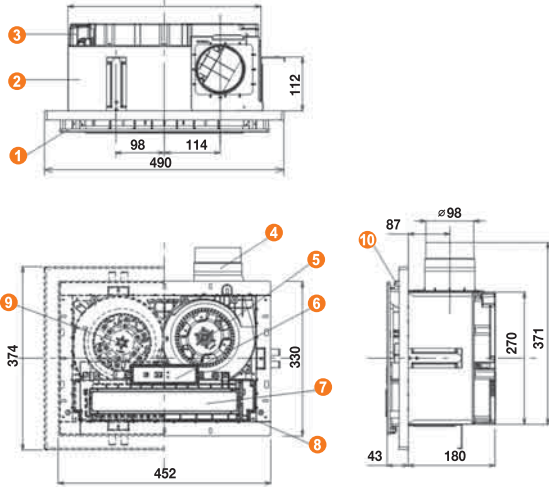
機身尺寸圖
