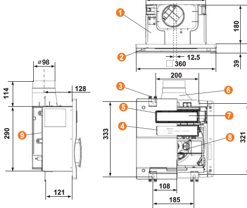
機身尺寸圖
